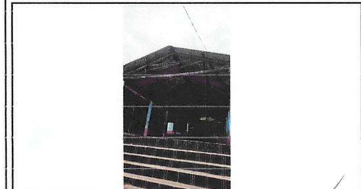
Foto 3: ESCENARIO Y AULA, Sustitución de estructura portante galvanizada y sustitucion de lamina por lamina troquelada aluzinc calibre 26
